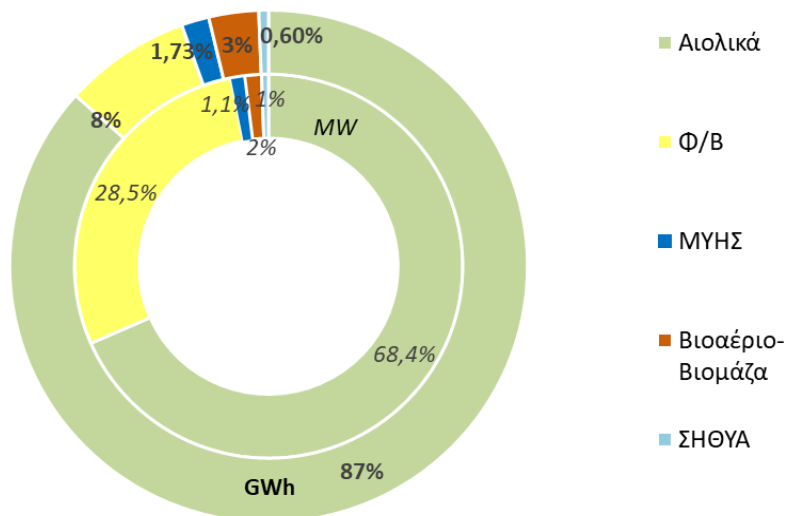
ΕΓΚΑΤΕΣΤΗΜΕΝΗ ΙΣΧΥΣ (MW) ΚΑΙ ΠΑΡΑΓΩΓΗ ΕΝΕΡΓΕΙΑΣ (GWh) ΜΟΝΑΔΩΝ ΣΕΔΠ - ΙΑΝΟΥΑΡΙΟΣ_2021
