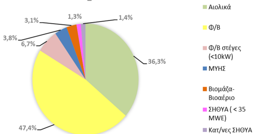
ΑΞΙΑ (%) ΑΝΑ ΤΕΧΝΟΛΟΓΙΑ ΑΠΕ & ΣΗΘΥΑ ΣΤΟ ΔΙΑΣΥΝΔΕΔΕΜΕΝΟ ΣΥΣΤΗΜΑ - ΑΠΡΙΛΙΟΣ_2020
