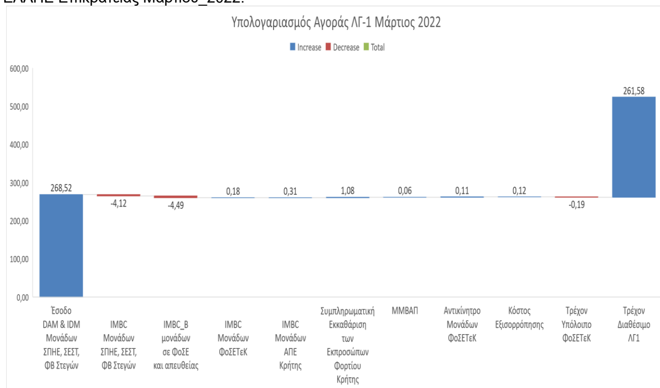
Διάγραμμα ανάλυσης της συνιστώσας «Τρέχον Διαθέσιμο ΛΓ-1» (Υπολογαριασμός Αγοράς) του ΕΛΑΠΕ Επικράτειας Μαρτίου_2022.
