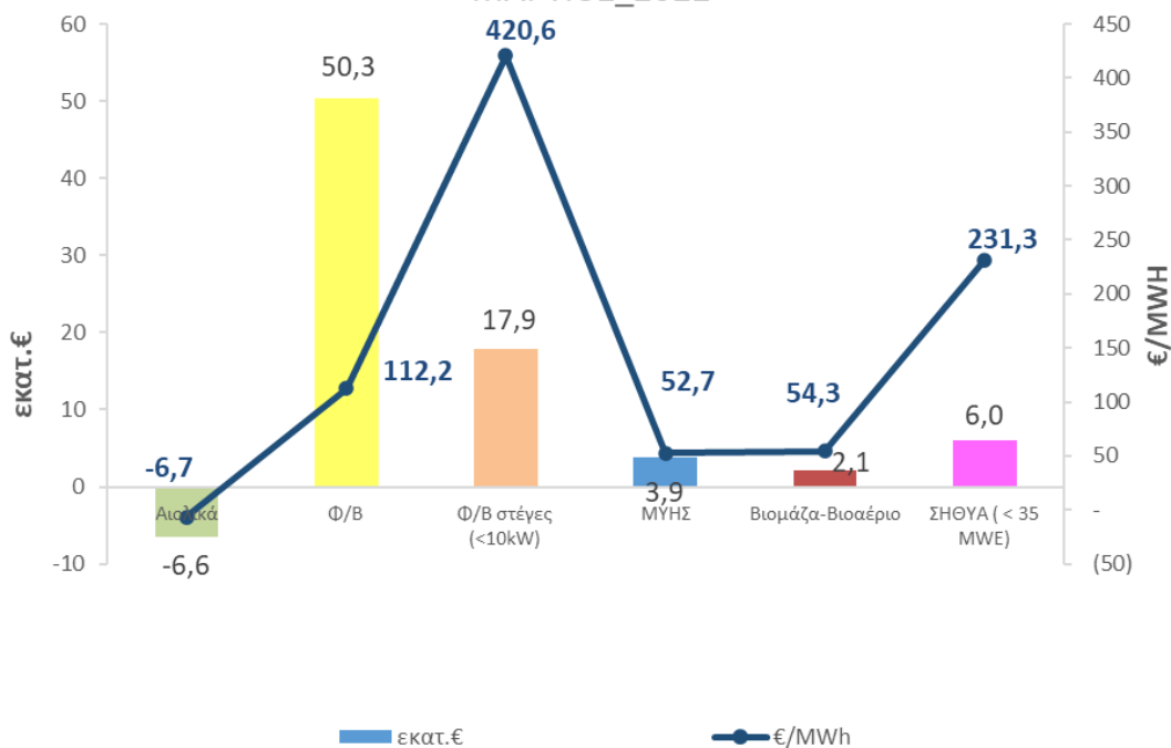
ΑΞΙΑ (εκατ. €) ΚΑΙ ΜΕΣΟΣΤΑΘΜΙΚΗ ΤΙΜΗ ΕΝΕΡΓΕΙΑΣ (€/MWh) ΑΠΕ & ΣΗΘΥΑ ΣΤΟ ΔΙΑΣΥΝΔΕΔΕΜΕΝΟ ΣΥΣΤΗΜΑ - ΜΑΡΤΙΟΣ_2022
