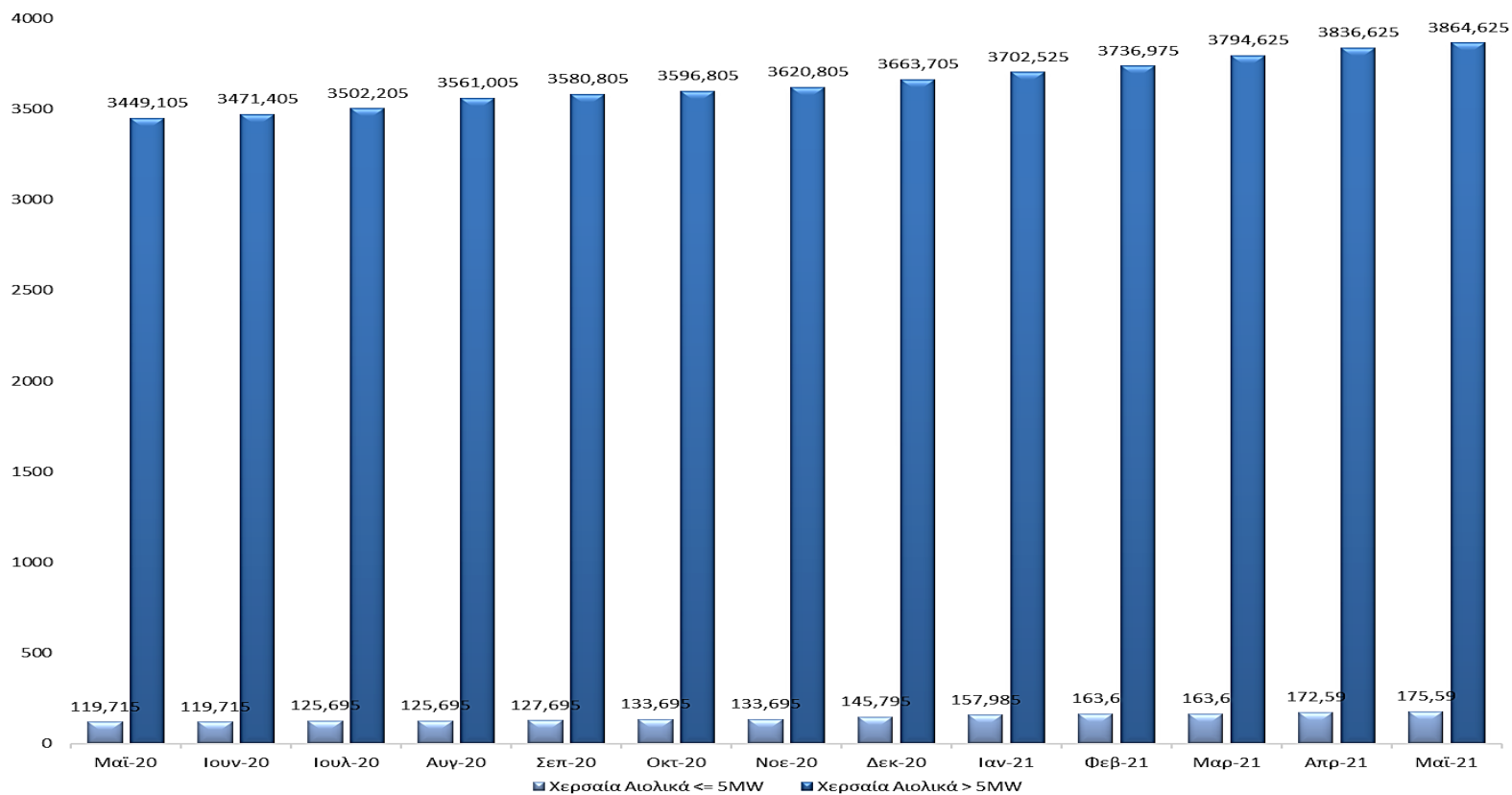
05_2021 ΓΕΩΓΡΑΦΙΚΗ ΚΑΤΑΝΟΜΗ & ΕΞΕΛΙΞΗ ΕΓΚΑΤΕΣΤΗΜΕΝΗΣ ΙΣΧΥΟΣ (MW) ΧΕΡΣΑΙΑ ΑΙΟΛΙΚΑ (Άρθρο 9 Ν.3468/2006)
