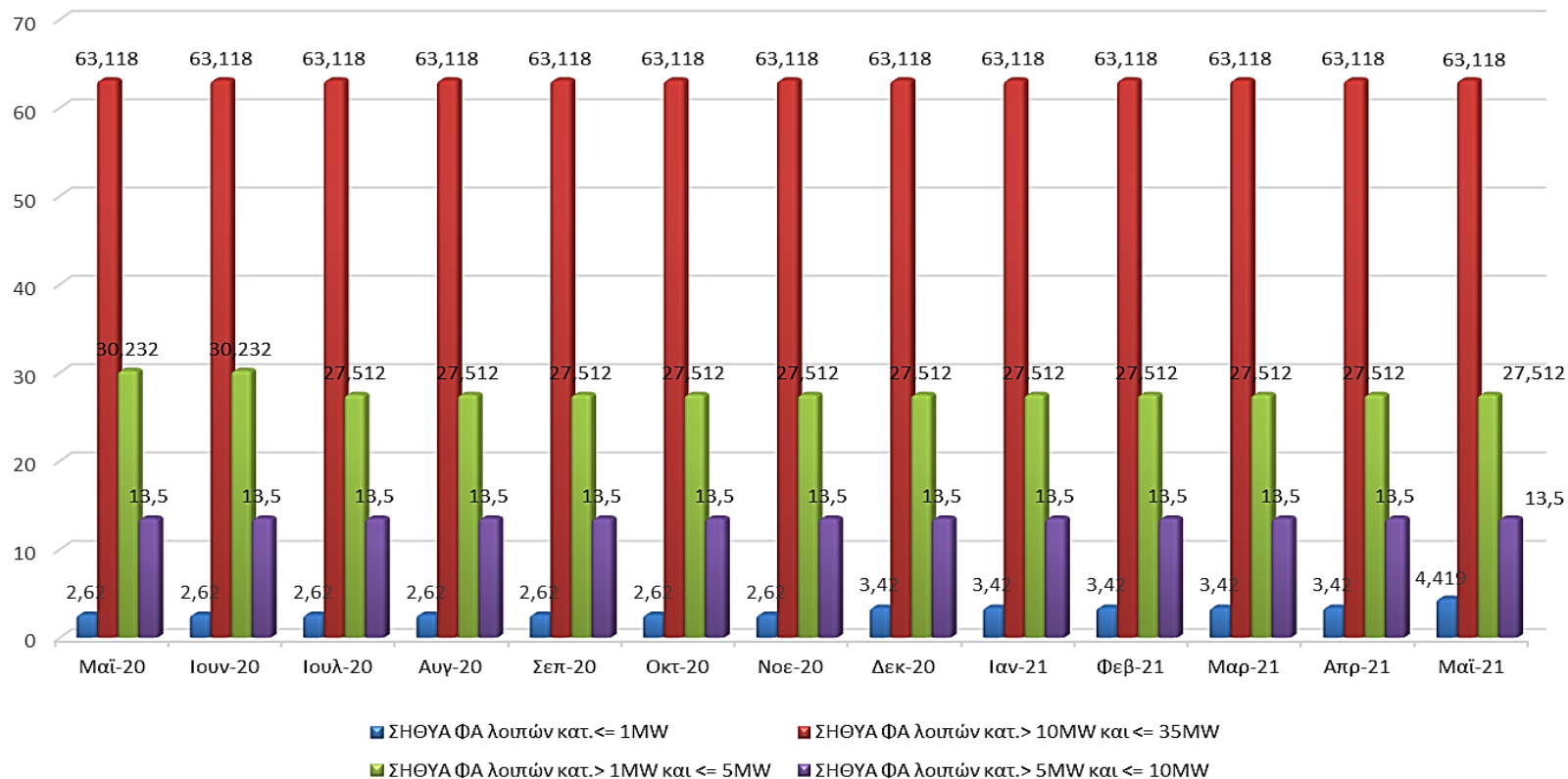
05_2021 ΓΕΩΓΡΑΦΙΚΗ ΚΑΤΑΝΟΜΗ & ΕΞΕΛΙΞΗ ΕΓΚΑΤΕΣΤΗΜΕΝΗΣ ΙΣΧΥΟΣ (MW) ΣΗΘΥΑ (Άρθρο 9 Ν.3468/2006)
