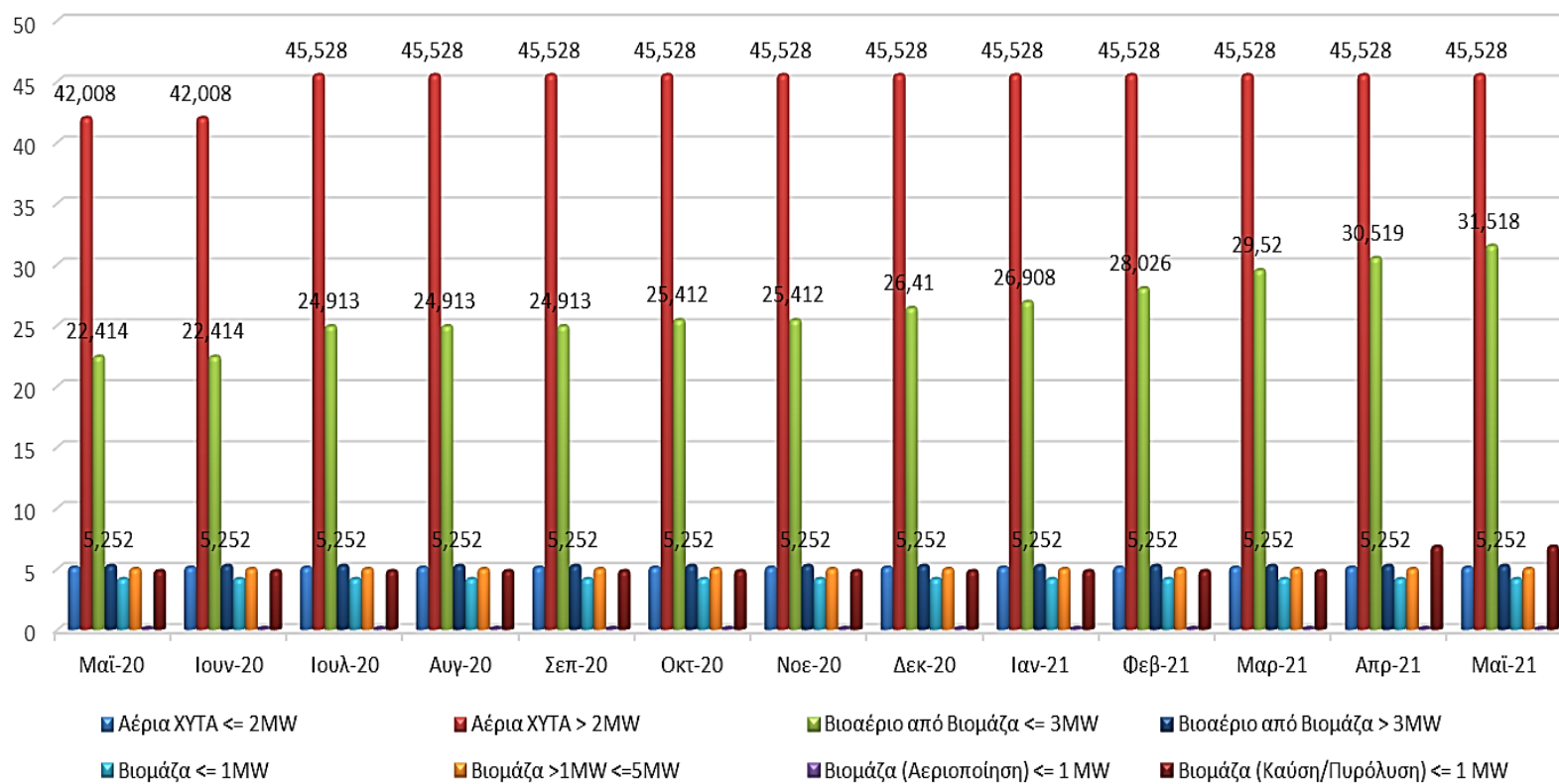
05_2021 ΓΕΩΓΡΑΦΙΚΗ ΚΑΤΑΝΟΜΗ & ΕΞΕΛΙΞΗ ΕΓΚΑΤΕΣΤΗΜΕΝΗΣ ΙΣΧΥΟΣ (MW) ΒΙΟΜΑΖΑ-ΒΙΟΑΕΡΙΟ (Άρθρο 9 Ν.3468/2006)
