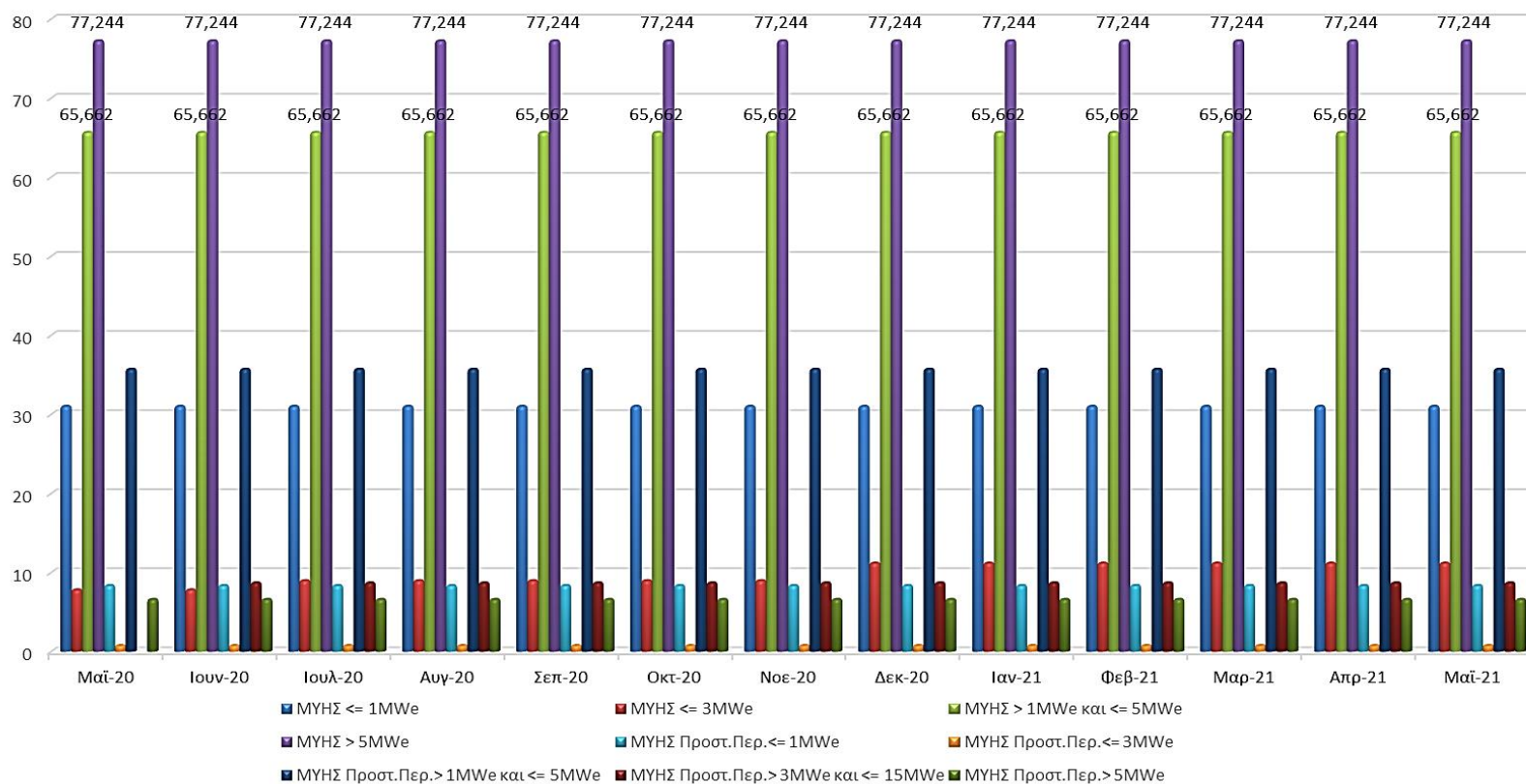
05_2021 ΓΕΩΓΡΑΦΙΚΗ ΚΑΤΑΝΟΜΗ & ΕΞΕΛΙΞΗ ΕΓΚΑΤΕΣΤΗΜΕΝΗΣ ΙΣΧΥΟΣ (MW) ΜΥΗΣ (Άρθρο 9 Ν.3468/2006)
