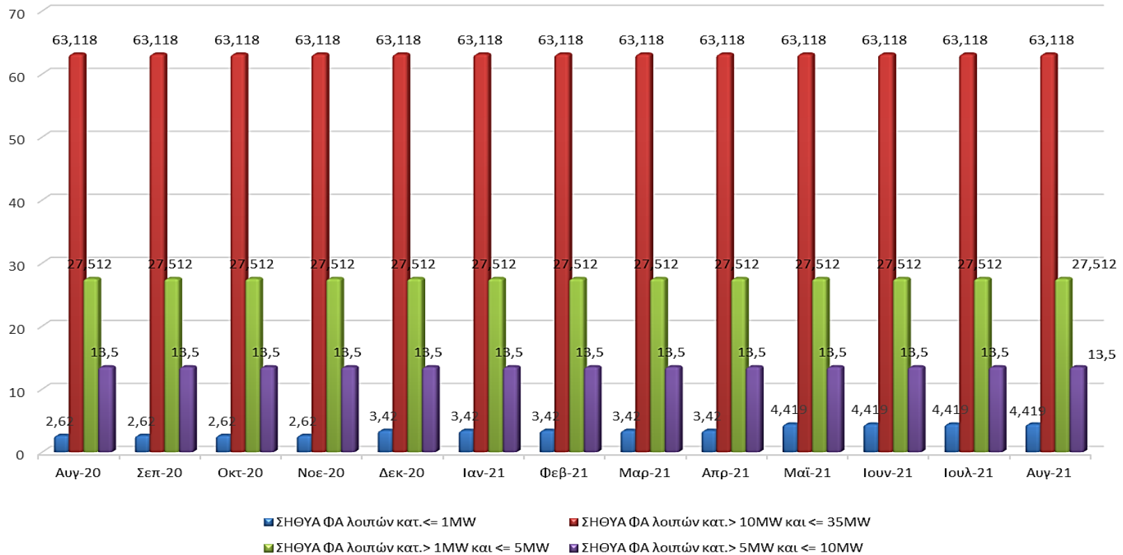
08_2021 ΓΕΩΓΡΑΦΙΚΗ ΚΑΤΑΝΟΜΗ & ΕΞΕΛΙΞΗ ΕΓΚΑΤΕΣΤΗΜΕΝΗΣ ΙΣΧΥΟΣ (MW) ΣΗΘΥΑ (Άρθρο 9 Ν.3468/2006)
