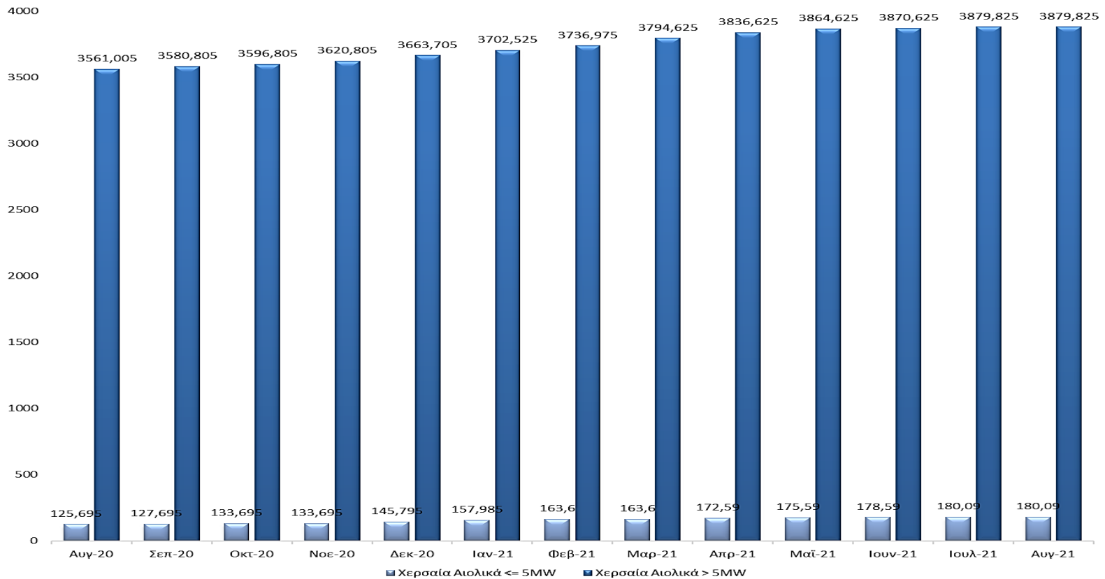
08_2021 ΓΕΩΓΡΑΦΙΚΗ ΚΑΤΑΝΟΜΗ & ΕΞΕΛΙΞΗ ΕΓΚΑΤΕΣΤΗΜΕΝΗΣ ΙΣΧΥΟΣ (MW) ΧΕΡΣΑΙΑ ΑΙΟΛΙΚΑ (Άρθρο 9 Ν.3468/2006)
