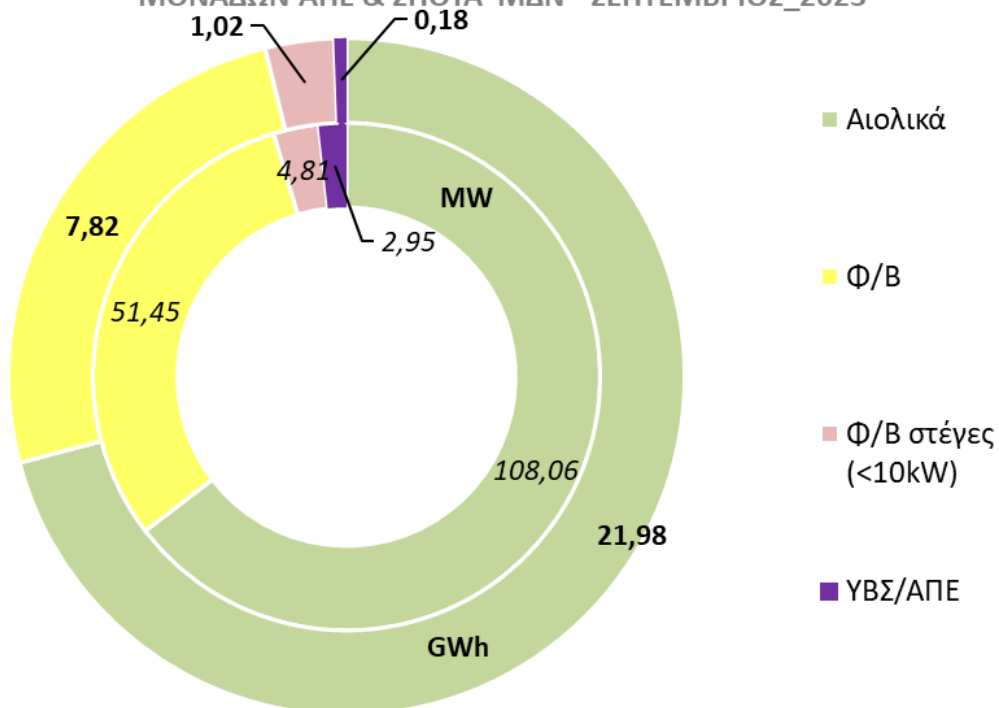
ΕΓΚΑΤΕΣΤΗΜΕΝΗ ΙΣΧΥΣ (MW) ΚΑΙ ΠΑΡΑΓΩΓΗ ΕΝΕΡΓΕΙΑΣ (GWh) ΜΟΝΑΔΩΝ ΑΠΕ & ΣΗΘΥΑ ΜΔΝ - ΣΕΠΤΕΜΒΡΙΟΣ_2023
