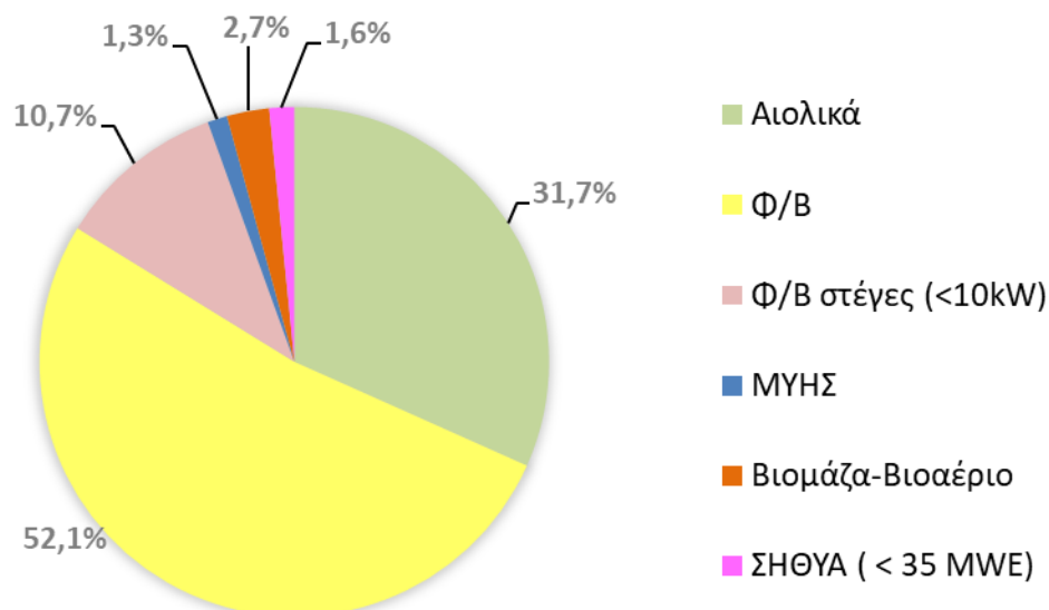
ΑΞΙΑ (%) ΑΝΑ ΤΕΧΝΟΛΟΓΙΑ ΜΟΝΑΔΩΝ ΑΠΕ & ΣΗΘΥΑ ΜΕ ΕΝΕΡΓΟΠΟΙΗΣΗ ΠΡΙΝ ΤΗΝ 1.1.2021 ΣΤΟ ΔΙΑΣΥΝΔΕΔΕΜΕΝΟ ΣΥΣΤΗΜΑ - ΑΥΓΟΥΣΤΟΣ_2023
