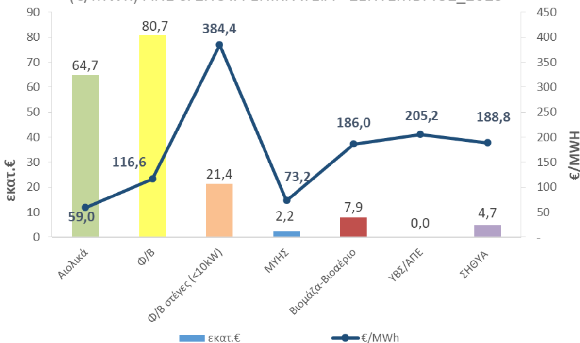
ΑΞΙΑ (εκατ. €) ΚΑΙ ΜΕΣΟΣΤΑΘΜΙΚΗ ΤΙΜΗ ΕΝΕΡΓΕΙΑΣ (€/MWh) ΑΠΕ & ΣΗΘΥΑ ΕΠΙΚΡΑΤΕΙΑ - ΣΕΠΤΕΜΒΡΙΟΣ_2023
