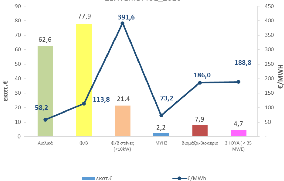
ΑΞΙΑ (εκατ. €) ΚΑΙ ΜΕΣΟΣΤΑΘΜΙΚΗ ΤΙΜΗ ΕΝΕΡΓΕΙΑΣ (€/MWh) ΑΠΕ & ΣΗΘΥΑ ΣΤΟ ΔΙΑΣΥΝΔΕΔΕΜΕΝΟ ΣΥΣΤΗΜΑ - ΣΕΠΤΕΜΒΡΙΟΣ_2023
