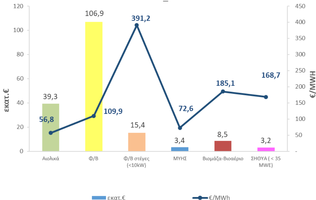
ΑΞΙΑ (εκατ. €) ΚΑΙ ΜΕΣΟΣΤΑΘΜΙΚΗ ΤΙΜΗ ΕΝΕΡΓΕΙΑΣ (€/MWh) ΑΠΕ & ΣΗΘΥΑ ΣΤΟ ΔΙΑΣΥΝΔΕΔΕΜΕΝΟ ΣΥΣΤΗΜΑ - ΙΟΥΛΙΟΣ_2023
