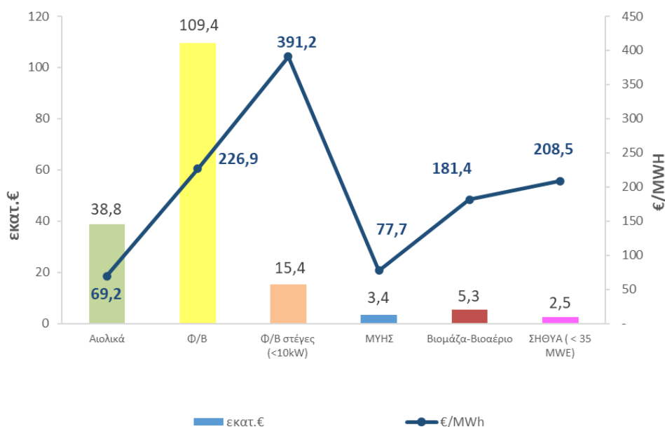
ΑΞΙΑ (εκατ. €) ΚΑΙ ΜΕΣΟΣΤΑΘΜΙΚΗ ΤΙΜΗ ΕΝΕΡΓΕΙΑΣ (€/MWh) ΜΟΝΑΔΩΝ ΑΠΕ & ΣΗΘΥΑ ΜΕ ΕΝΕΡΓΟΠΟΙΗΣΗ ΠΡΙΝ ΤΗΝ 1.1.2021 ΣΤΟ ΔΙΑΣΥΝΔΕΔΕΜΕΝΟ ΣΥΣΤΗΜΑ - ΙΟΥΛΙΟΣ_2023
