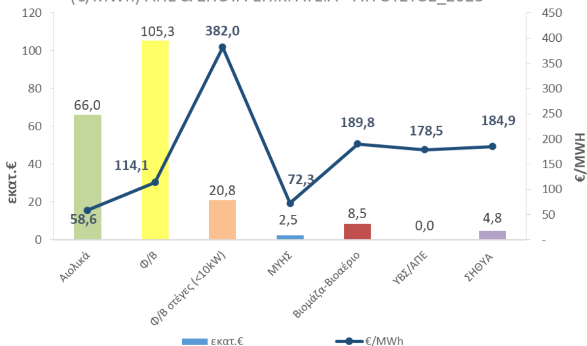
ΑΞΙΑ (εκατ. €) ΚΑΙ ΜΕΣΟΣΤΑΘΜΙΚΗ ΤΙΜΗ ΕΝΕΡΓΕΙΑΣ (€/MWh) ΑΠΕ & ΣΗΘΥΑ ΕΠΙΚΡΑΤΕΙΑ - ΑΥΓΟΥΣΤΟΣ_2023
