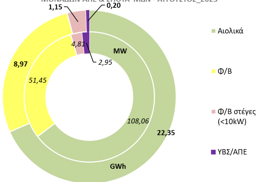
ΕΓΚΑΤΕΣΤΗΜΕΝΗ ΙΣΧΥΣ (MW) ΚΑΙ ΠΑΡΑΓΩΓΗ ΕΝΕΡΓΕΙΑΣ (GWh) ΜΟΝΑΔΩΝ ΑΠΕ & ΣΗΘΥΑ ΜΔΝ - ΑΥΓΟΥΣΤΟΣ_2023
