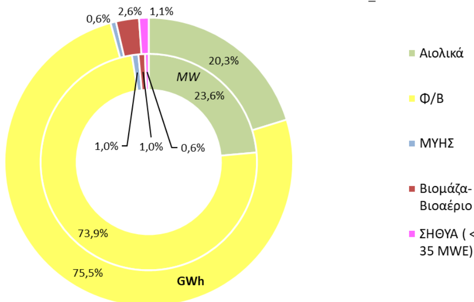
ΕΓΚΑΤΕΣΤΗΜΕΝΗ ΙΣΧΥΣ (MW) ΚΑΙ ΠΑΡΑΓΩΓΗ ΕΝΕΡΓΕΙΑΣ (GWh) ΜΟΝΑΔΩΝ ΑΠΕ & ΣΗΘΥΑ ΜΕ ΕΝΕΡΓΟΠΟΙΗΣΗ ΜΕΤΑ ΤΗΝ 1.1.2021 ΣΤΟ ΔΙΑΣΥΝΔΕΔΕΜΕΝΟ ΣΥΣΤΗΜΑ - ΙΟΥΛΙΟΣ_2023
