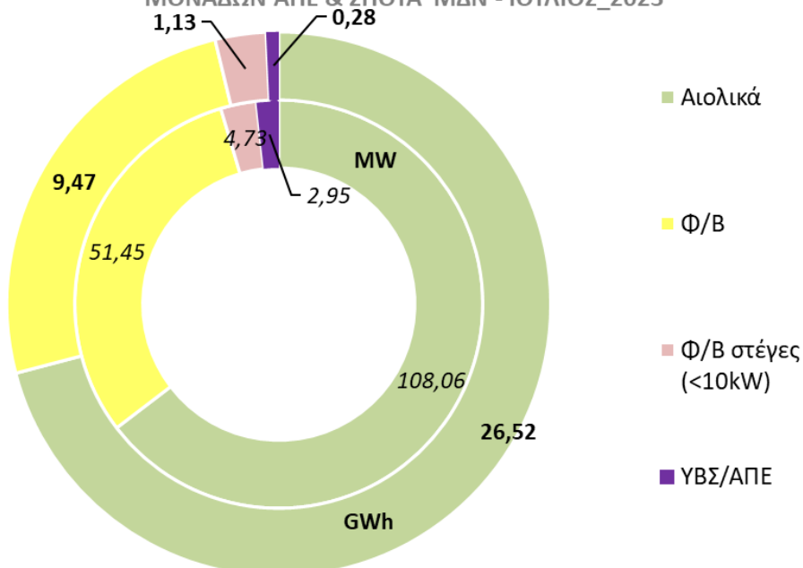
ΕΓΚΑΤΕΣΤΗΜΕΝΗ ΙΣΧΥΣ (MW) ΚΑΙ ΠΑΡΑΓΩΓΗ ΕΝΕΡΓΕΙΑΣ (GWh) ΜΟΝΑΔΩΝ ΑΠΕ & ΣΗΘΥΑ ΜΔΝ - ΙΟΥΛΙΟΣ_2023
